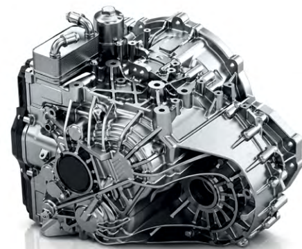
7-ступенчатая коробка передач с двойным сцеплением «мокрого» типа
